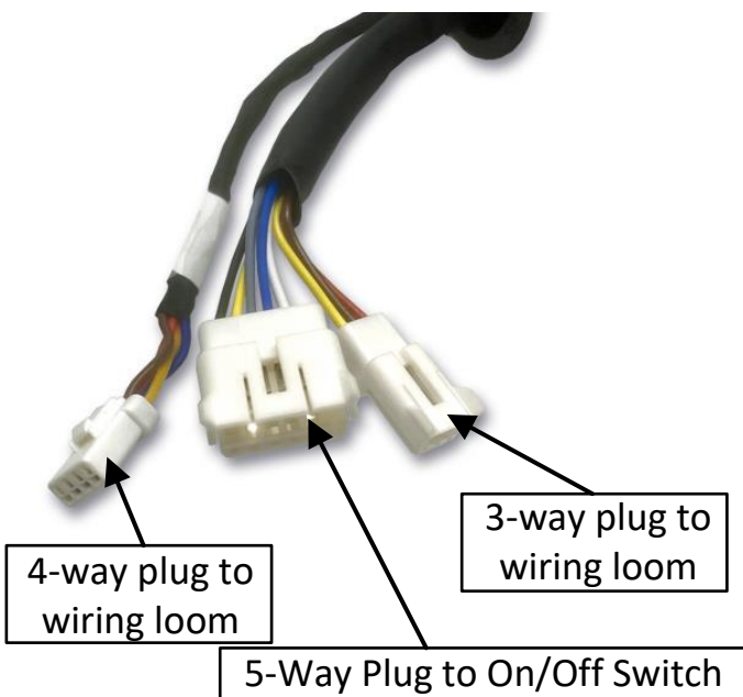
2A) Timer Box Connections
